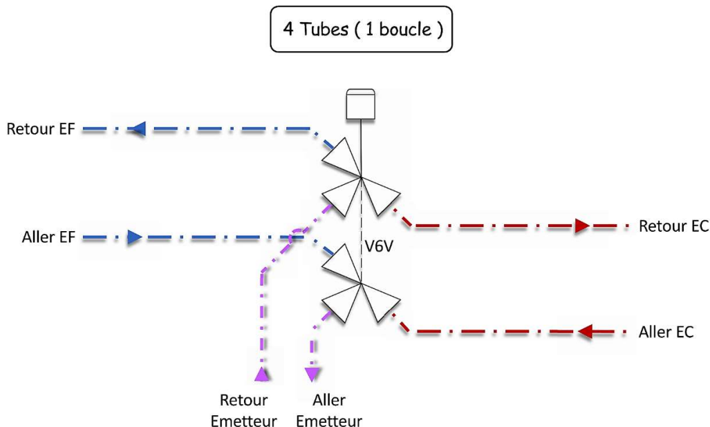
Schéma hydraulique
